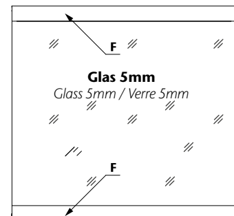
Türe ohne vertikalem Rahmen Door without vertical frame / Porte sans à encadrement vertical
