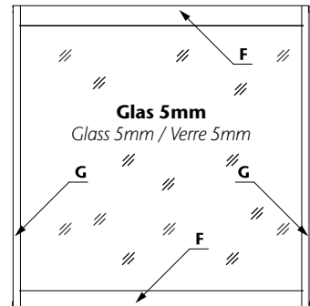
Türe mit vertikalem Rahmen Door with vertical frame / Porte à encadrement vertical
